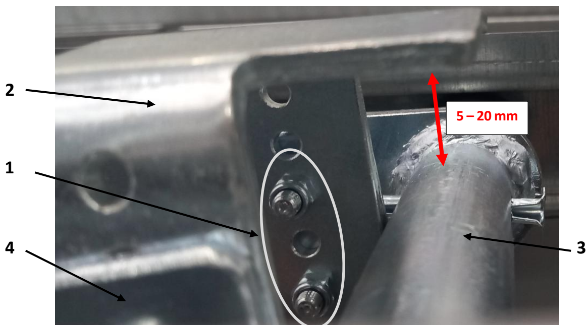
Rys. 27 Regulacja wysokości haka ryglującego w klapach o szerokości otworu wylotowego \geq 130 cm.
