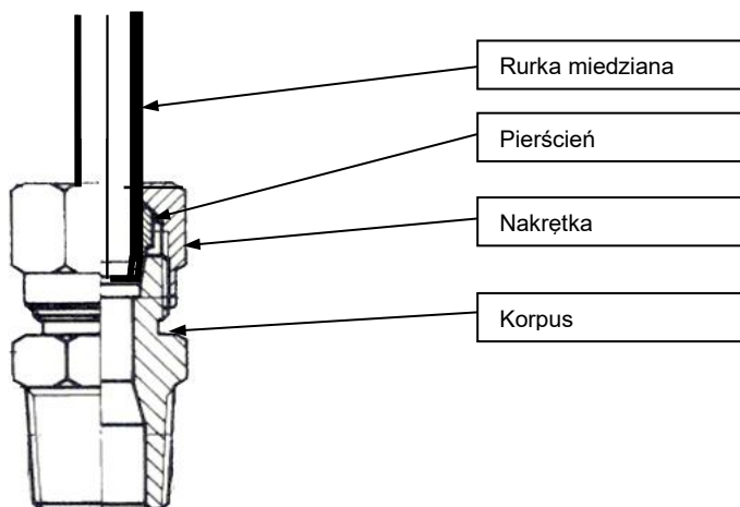
Rys. 28 Połączenie śrubunku z rurką miedzianą/stalową.
