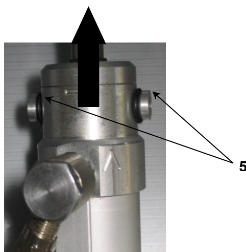
Rys. 35 Siłownik pneumatyczny PUAV – kierunek zwalniania rygla.
