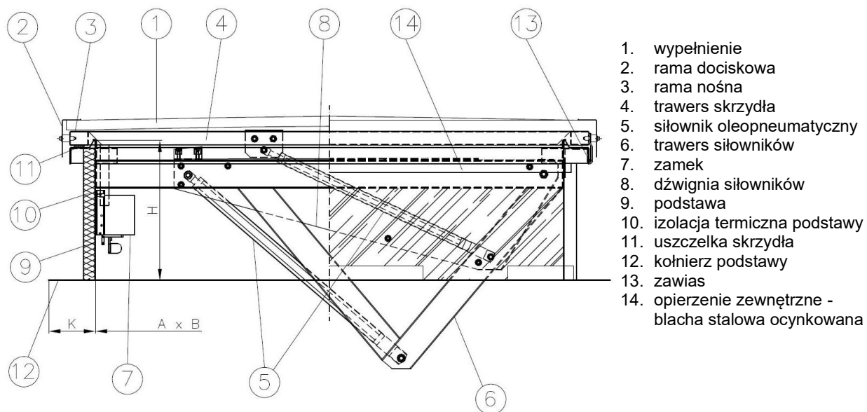
Rys. 1 Przekroje poprzeczne kłap mcr PROLIGHT
