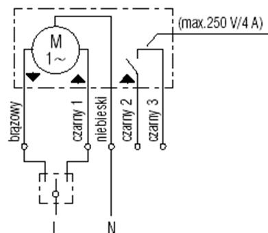
Rys. 42 Siłownik JMBB-500-300-LA.
