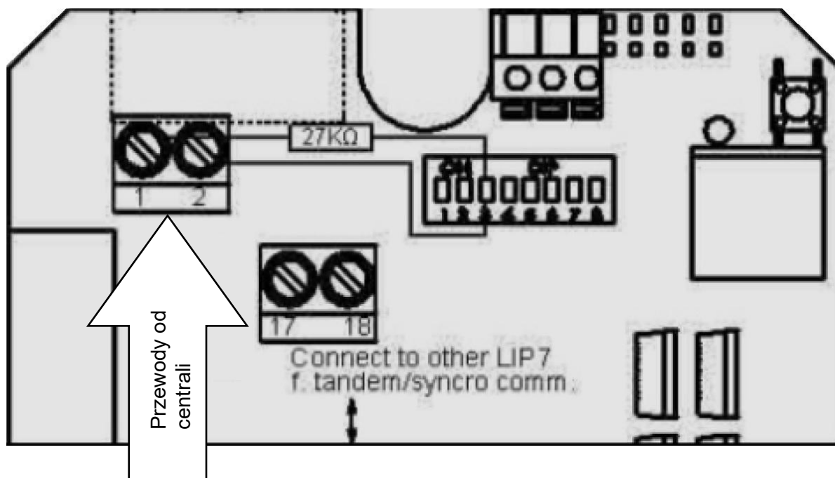
Rys. 37 Zaciski do podłączenia instalacji sterującej – zacisk 1 i zacisk 2.
