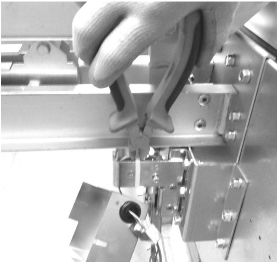
Rys. 46 Przecinanie opaski zaciskowej w celu odbezpieczenia zamka.
